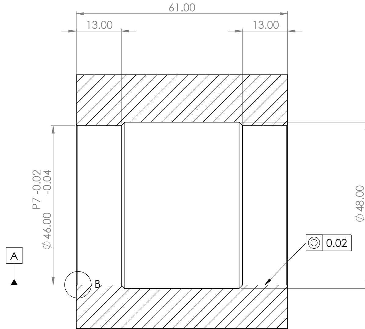
SECTION A-A
